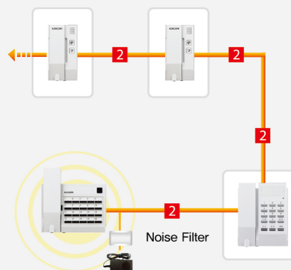
TYPE 4 모자식 인터폰
