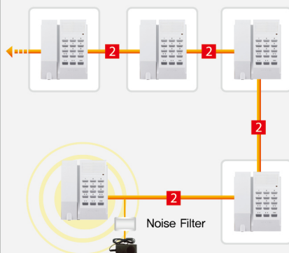
TYPE 3 상호식 인터폰 + 키폰타입
