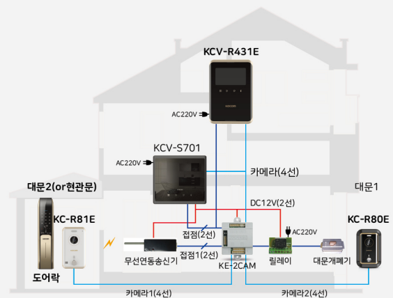
주택 · 빌라 · 단독주택 (출입구 2곳)
