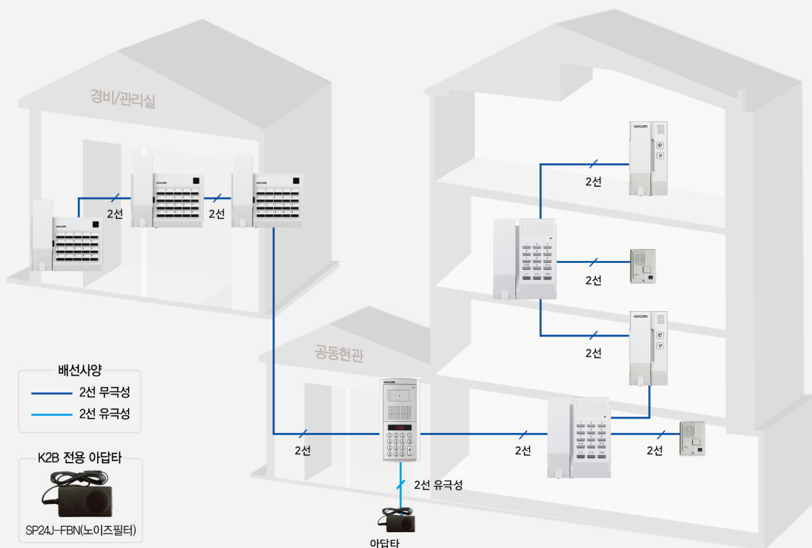
TYPE 2 상호식 인터폰
