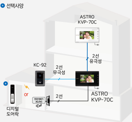
2층 주택 (2선식)
