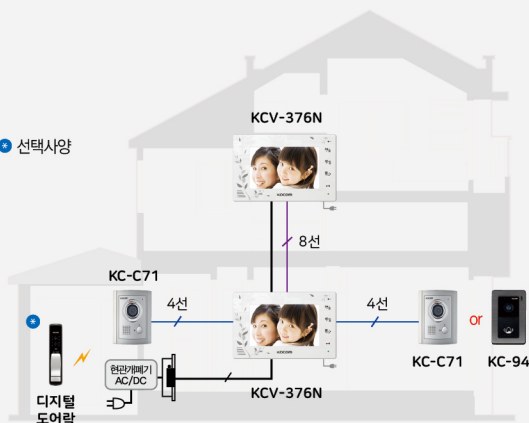
주택 · 빌라 · 단독주택 (출입구 2곳)
